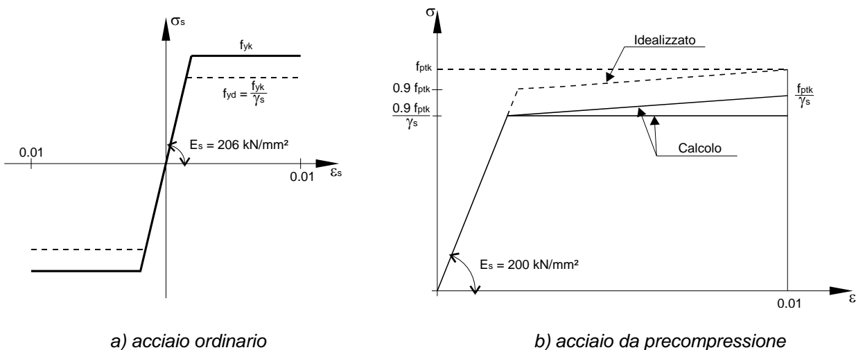
Fig. 3 - Diagramma di calcolo \sigma - \varepsilon
