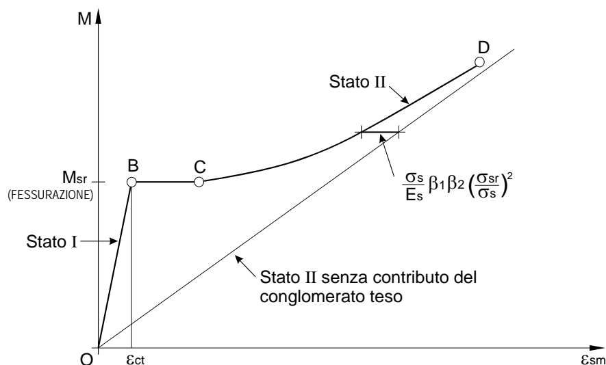
Fig. 6 - Diagramma M - \varepsilon_{sm}
