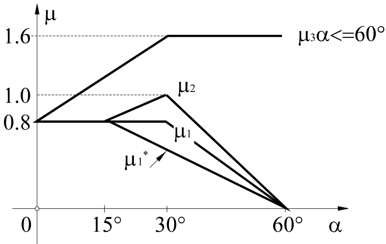
Fig. 6.2 - Coefficienti di forma per coperture a falde
